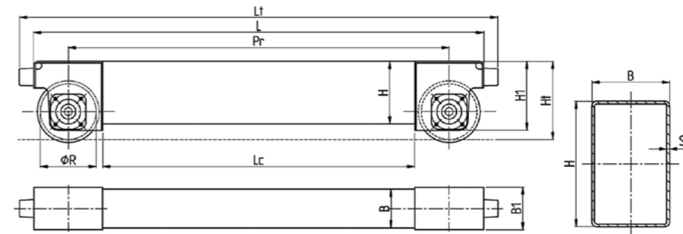
Conjunto cabezal
